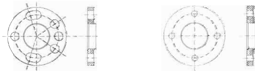
Ausführung D
